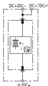
Prinzipschaltbild
