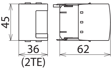
Maßbild
