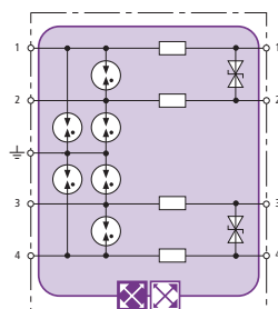
Prinzipschaltbild
