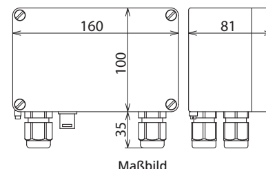
Maßbild
