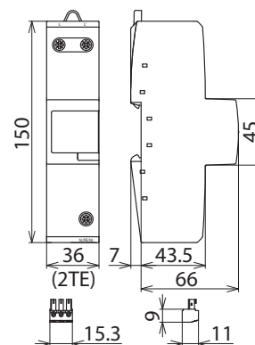
Maßbild
