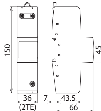
Maßbild
