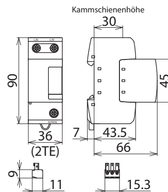
Maßbild
