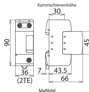
Maßbild
