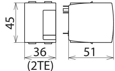
Maßbild
