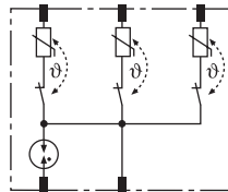
Prinzipschaltbild
