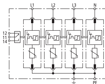
Prinzipschaltbild
