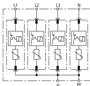
Prinzipschaltbild
