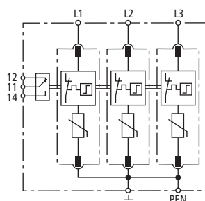
Prinzipschaltbild
