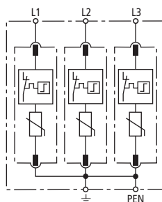
Prinzipialschaltbild
