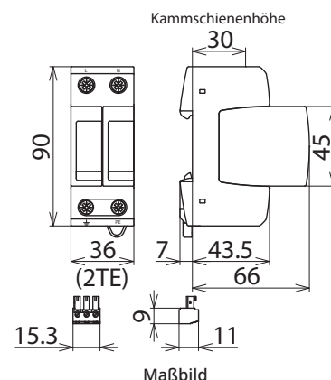
Maßbild
