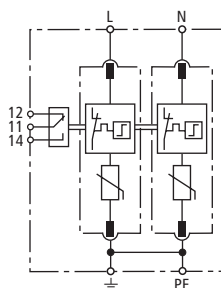
Prinzipschaltbild
