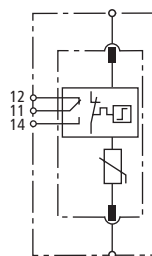
Prinzipialschaltbild
