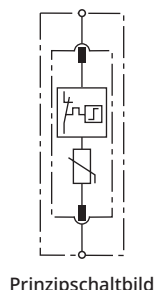
Prinzipschaltbild
