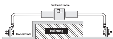
Prinzipschaltbild
