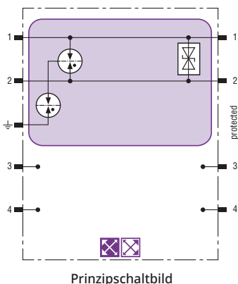
Prinzipschaltbild
