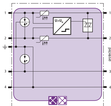
Prinzipschaltbild
