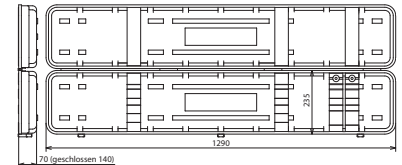
Maßbild
