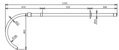
Maßbild
