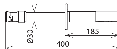
Maßbild
