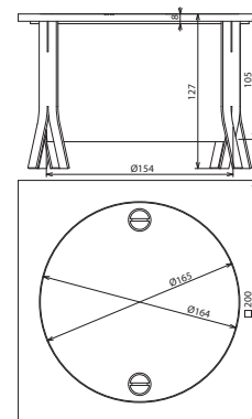
Maßbild
