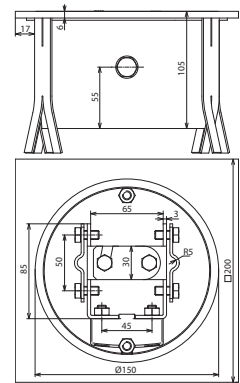
Maßbild
