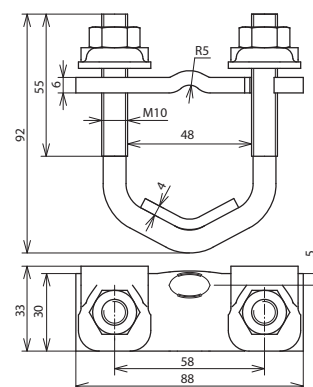
Maßbild
