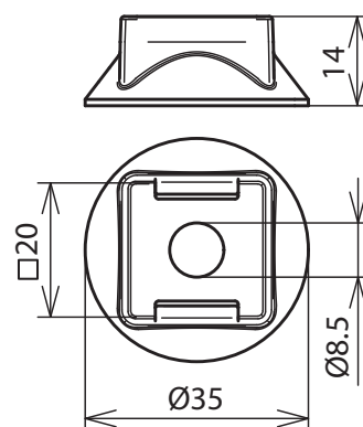
Maßbild
