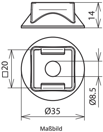
Maßbild
