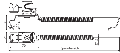
Maßbild
