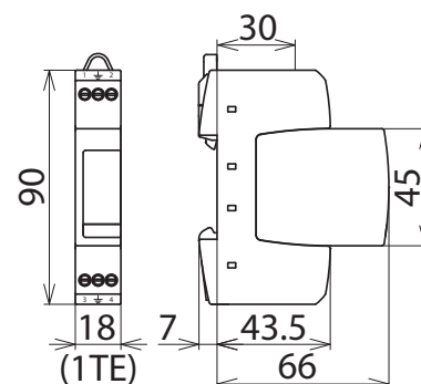
Maßbild
