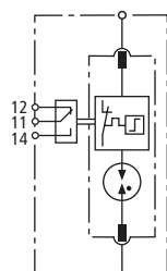
Prinzipschaltbild
