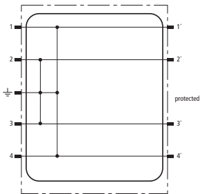
Prinzipschaltbild
