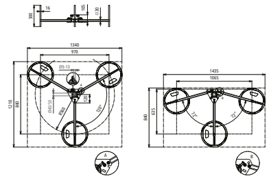
Maßbild
