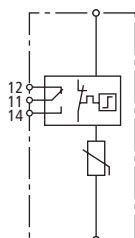
Prinzipschaltbild
