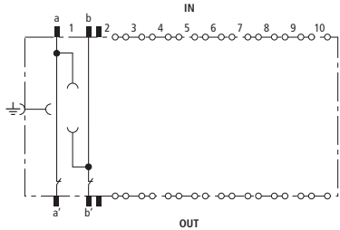
Prinzipschaltbild
