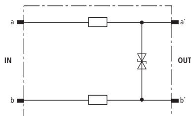
Prinzipschaltbild
