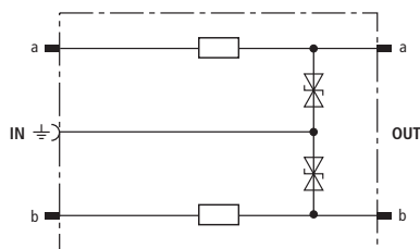
Prinzipschaltbild
