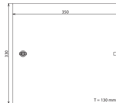
Maßbild
