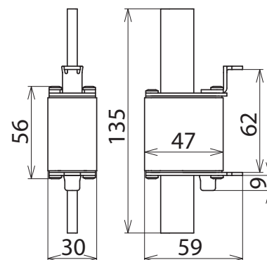
Maßbild
