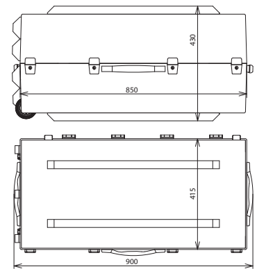
Maßbild
