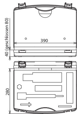
Maßbild
