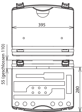
Maßbild
