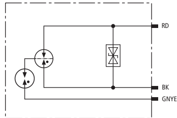
Prinzipschaltbild
