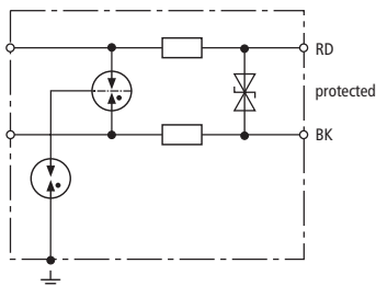
Prinzipschaltbild
