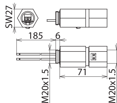
Maßbild
