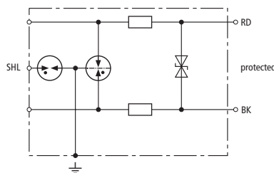
Prinzipschaltbild
