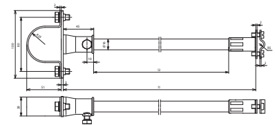
Maßbild
