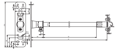
Maßbild
