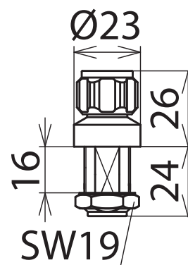
Maßbild
