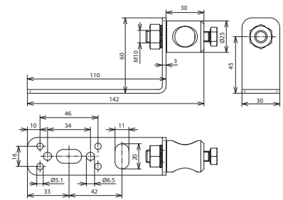
Maßbild
