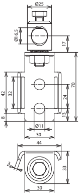
Maßbild
