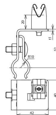
Maßbild
