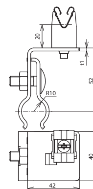
Maßbild
